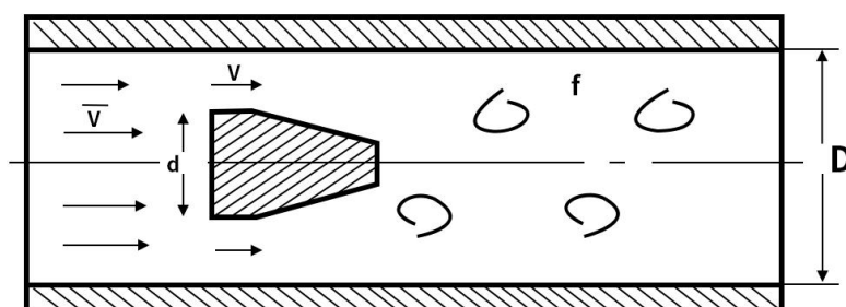
图一 圆管内的涡街
