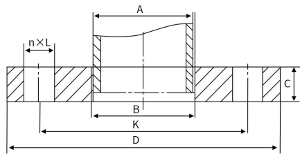
平面 (FF) 板式平焊钢制管法兰
