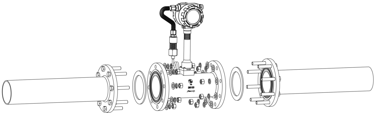
法兰连接示意图
