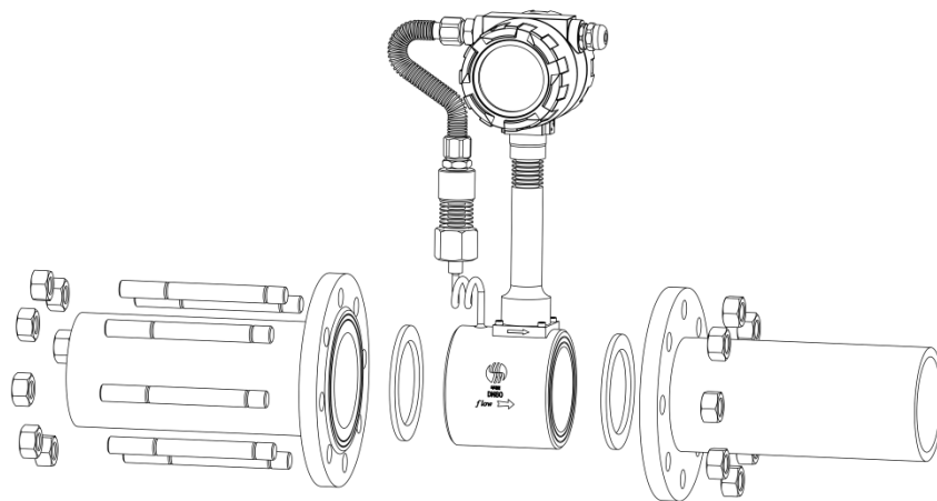
夹持式涡街流量计安装示意图
