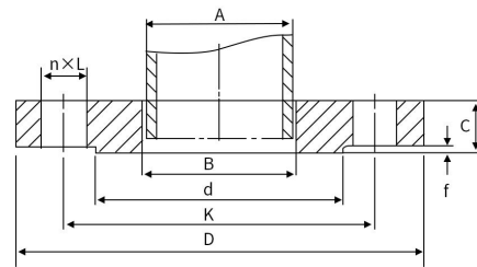
突面 (RF) 板式平焊钢制管法兰
